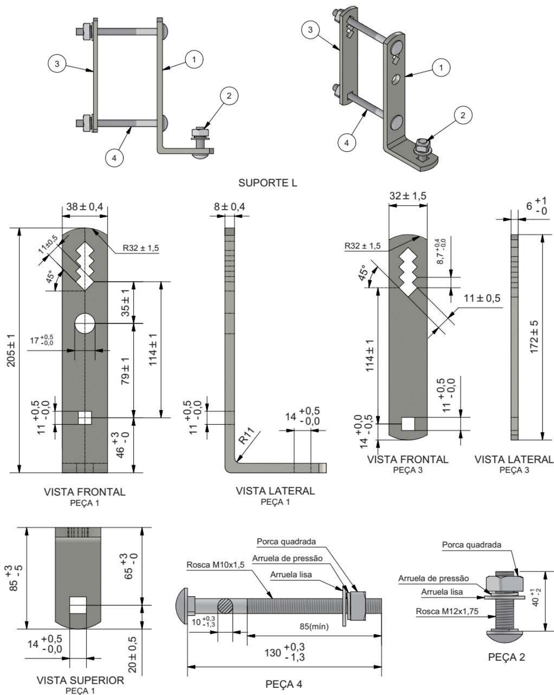
Figura 1 - Suporte L
